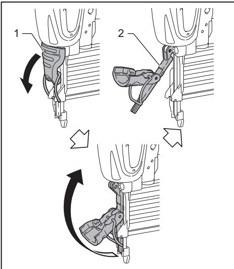
► 1. Latch 2. Door
